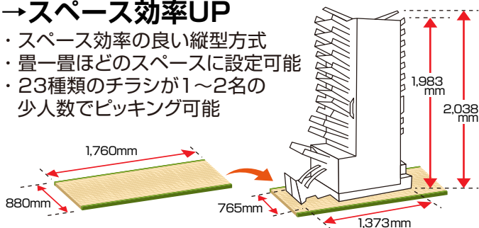
■ DM-A230Si・DM-230Si (折り棚バーコードキット未装着時) (紙受ユニット装着時)
